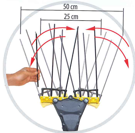
SPOSTAMENTO PETTINE. RAKE MOVEMENT DEPLACEMENT PEIGNES DESPLAZAMIENTO PEINE
